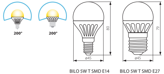
BILO 5W T SMD E14
